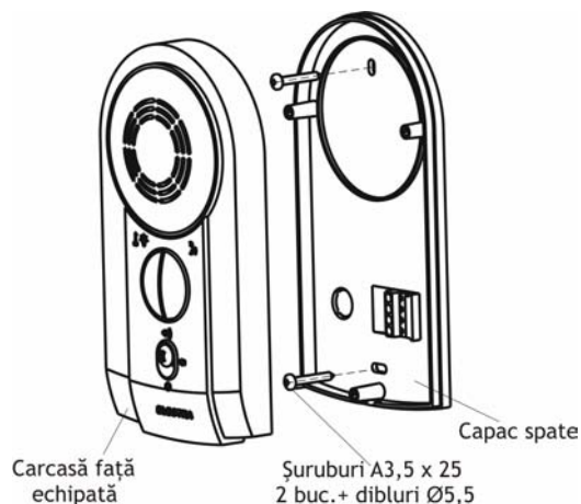
Fig. 1 Instalarea postului interior audio IA 02
