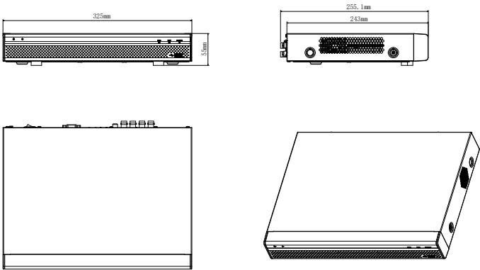
DHI-XVR5116HE-S2
